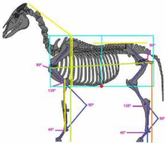
Afb. 3: Het evenwichtsmodel geprojecteerd op het paardenskelet. De lichtblauwe lijnen geven het rechthoeksmodel weer, te verdelen in twee vierkanten, met middenonder het diepste punt van de romp (de rode stip). De gele lijnen tonen de lengte van de voorbenen en de rompdiepte, de groene lijnen wijzen op de romplengte en de schofthoogte. De oranje lijn vormt de loodlijn die vanaf zitbeen, langs pijpbeen, pal achter de hoof hoort te eindigen. De donkerblauwe lijnen verduidelijken de hoeken die de dragende gewrichten behoren te maken.
